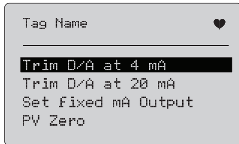
图 35. 微调、设置及归零屏幕
