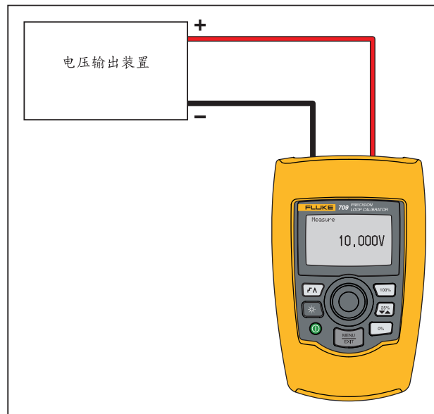
图 8. 电压测量连接
