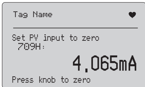
图 39. PV 归零屏幕
