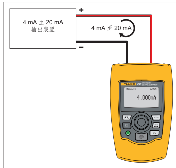
图 6. mA 测量连接
