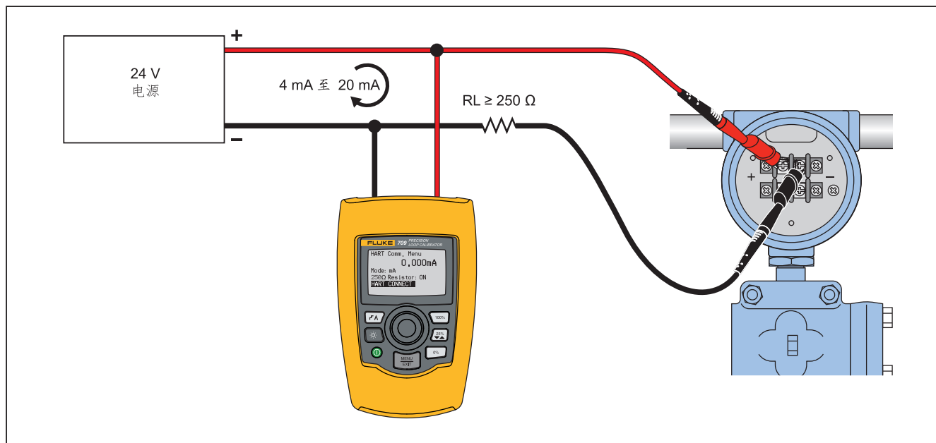
图 22. 位于电路之间，仅限通信器连接
