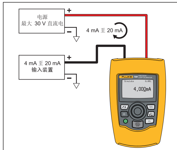
图 5. mA 模拟连接
