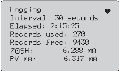
图 47. 活动日志屏幕
