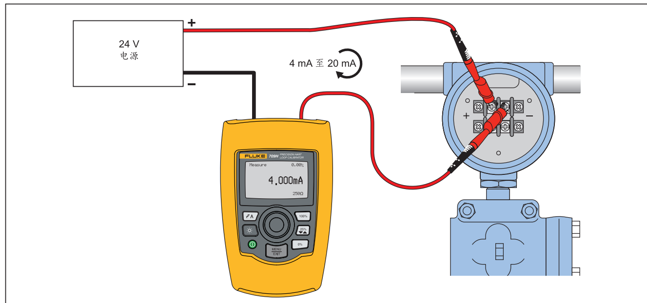
图 20. 位于电路之中，外部回路电源
