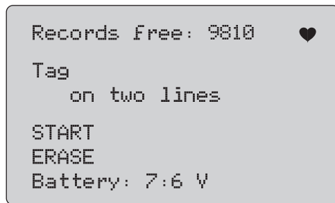
图 45. 数据日志屏幕
