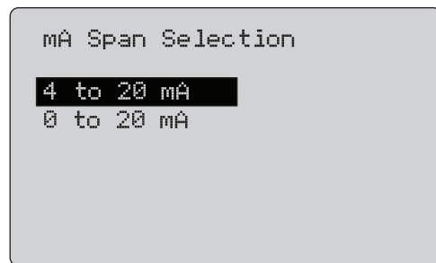
图 15. mA 跨度选择屏幕
