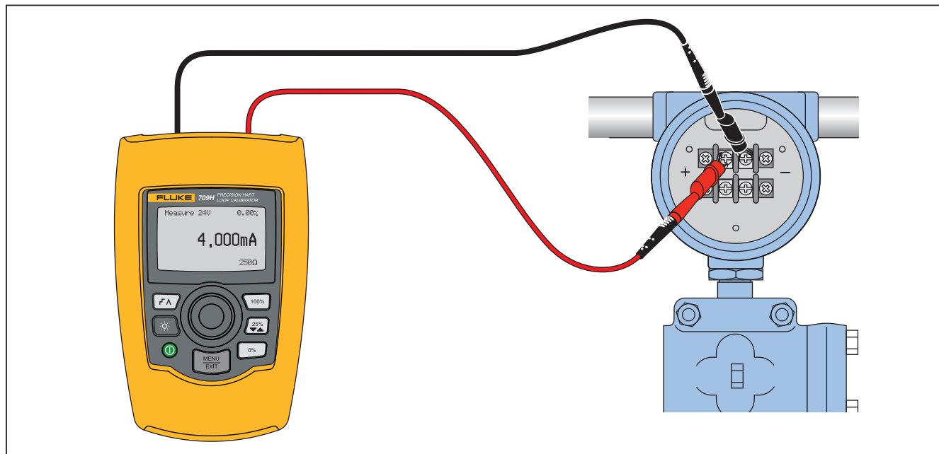
图 21. 位于电路之中，709H 回路电源
