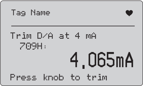
图 36. 4 mA 微调屏幕
