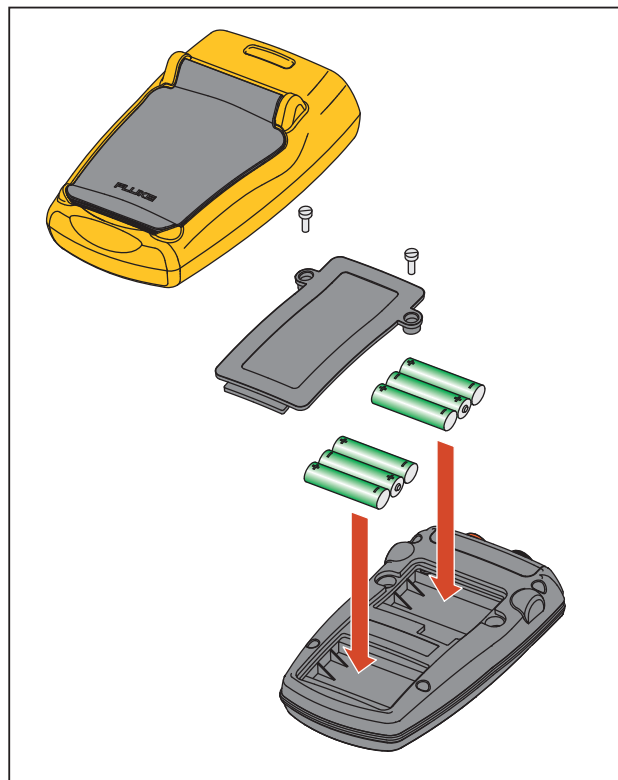
图 48. 更换电池
