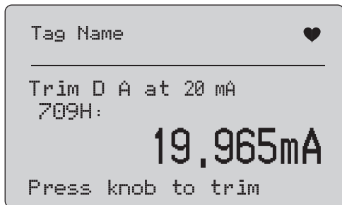
图 37. 20 mA 微调屏幕
