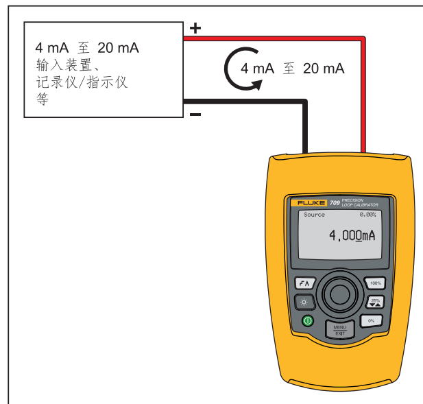
图 4. mA 输出连接
