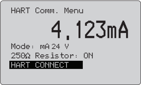
图 23. HART Comm. Menu（HART 通信菜单）屏幕
