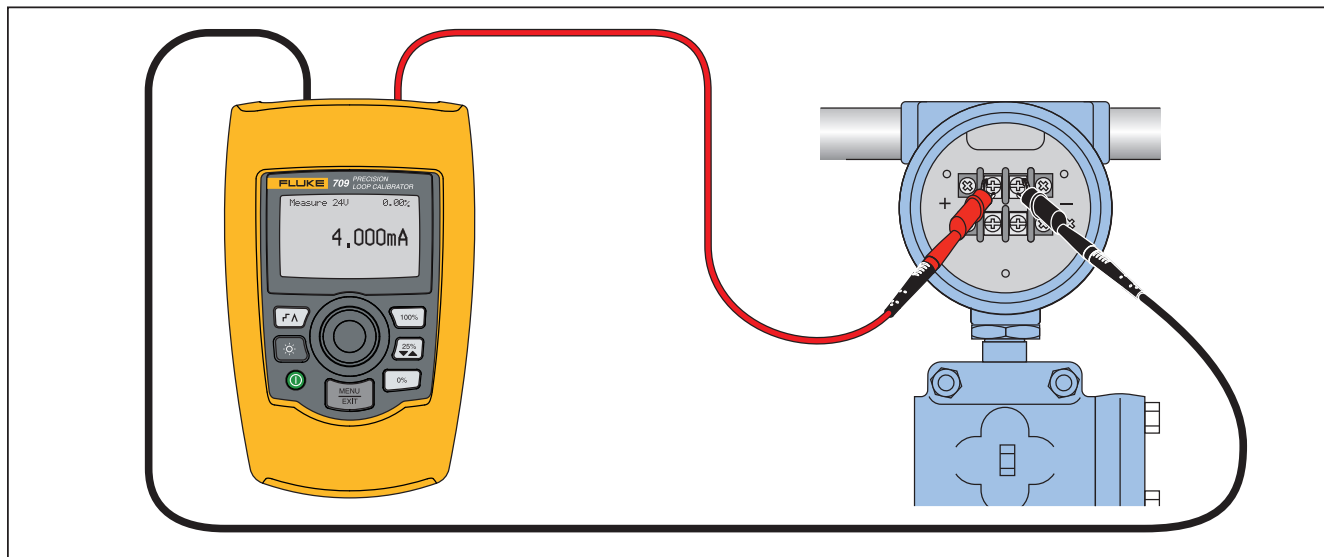
图 7. 24 V 电压下 mA 测量连接
