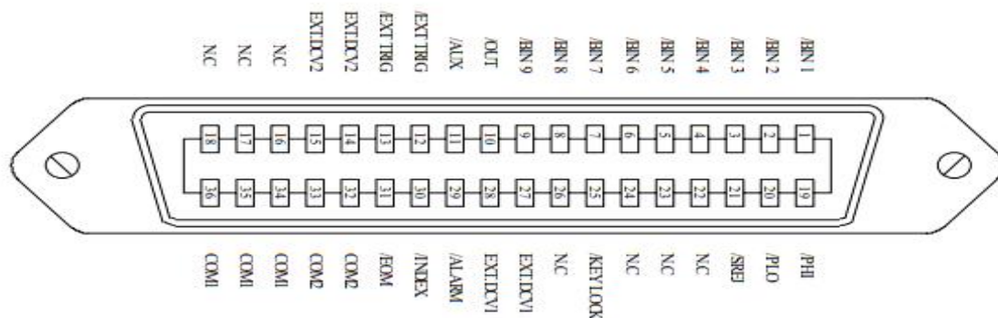
Handler 接口管脚定义
