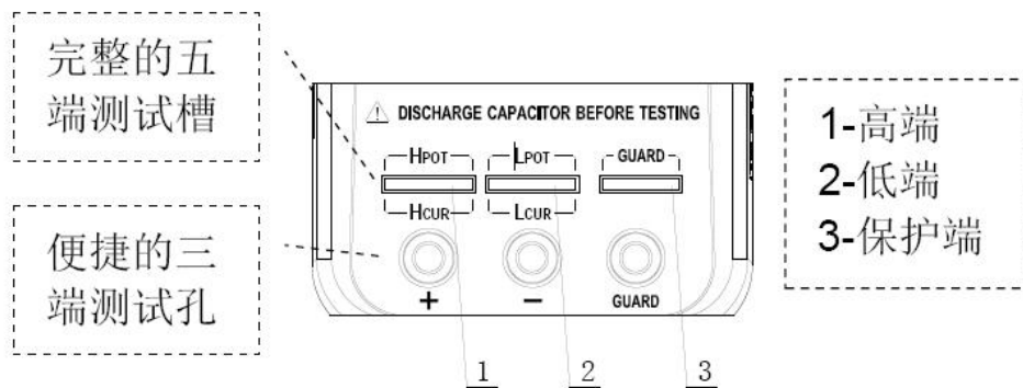
图 4 测试端口
