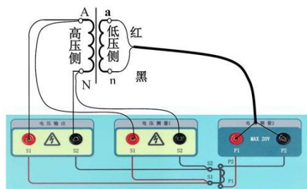
⑦ PT变比极性测量方案
