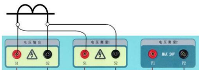
③ CT绕组直流电阻测量方案
