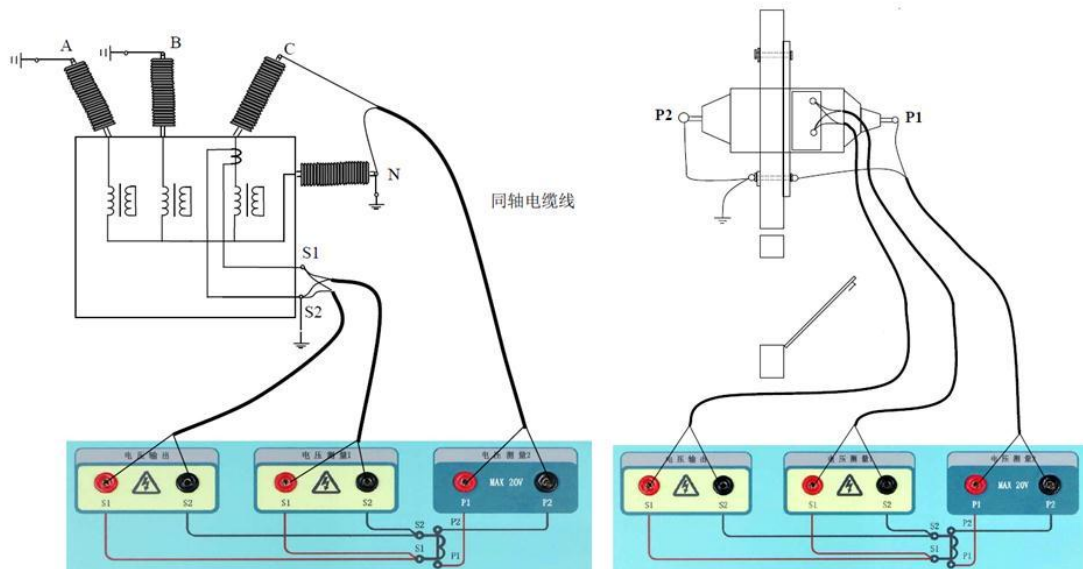
③ 穿墙安装 CT 接线。
