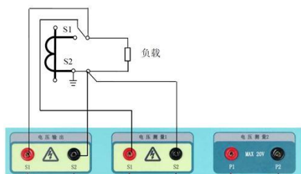
⑤ CT二次回路负载测量方案
