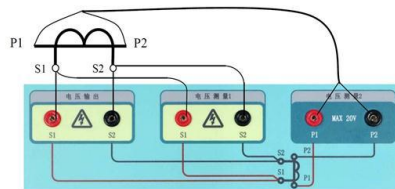
② CT变比极性、比差角差测量方案
