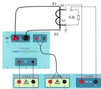
④ CT升流保持 (使用外置升流器) 测量方案 3
