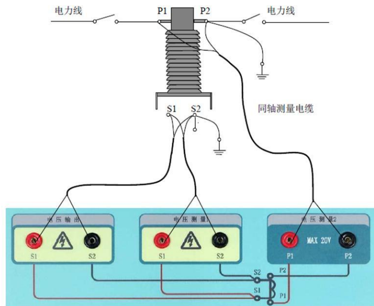
① 常规安装 CT 接线
