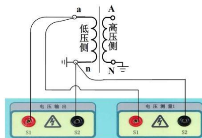
⑧ PT绕组直流电阻测量方案
