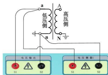
⑥ PT励磁特性测量方案
