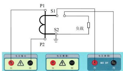
④ CT升流保持 (使用内置电源) 测量方案 2
