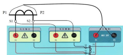
① CT励磁特性、变比、极性、直流电阻测量方案
