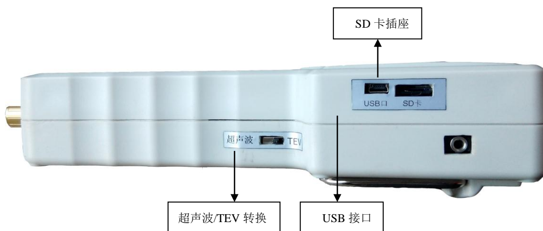
主机侧面图
