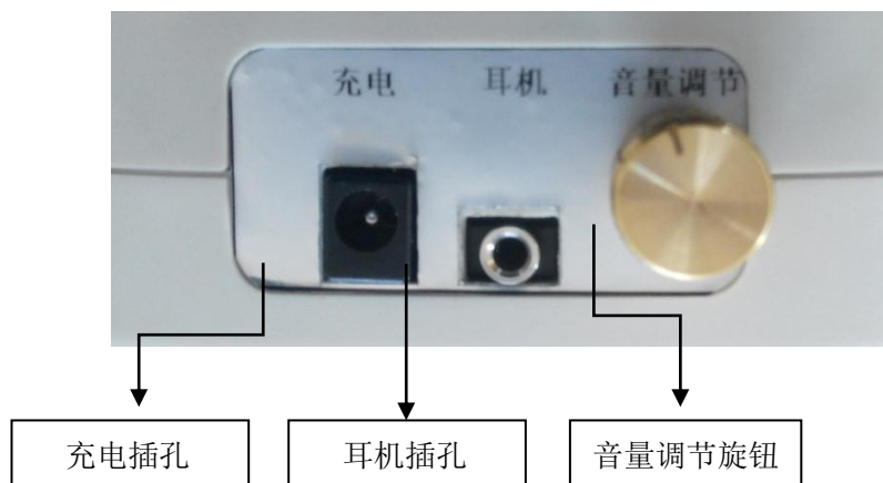
主机底面图
