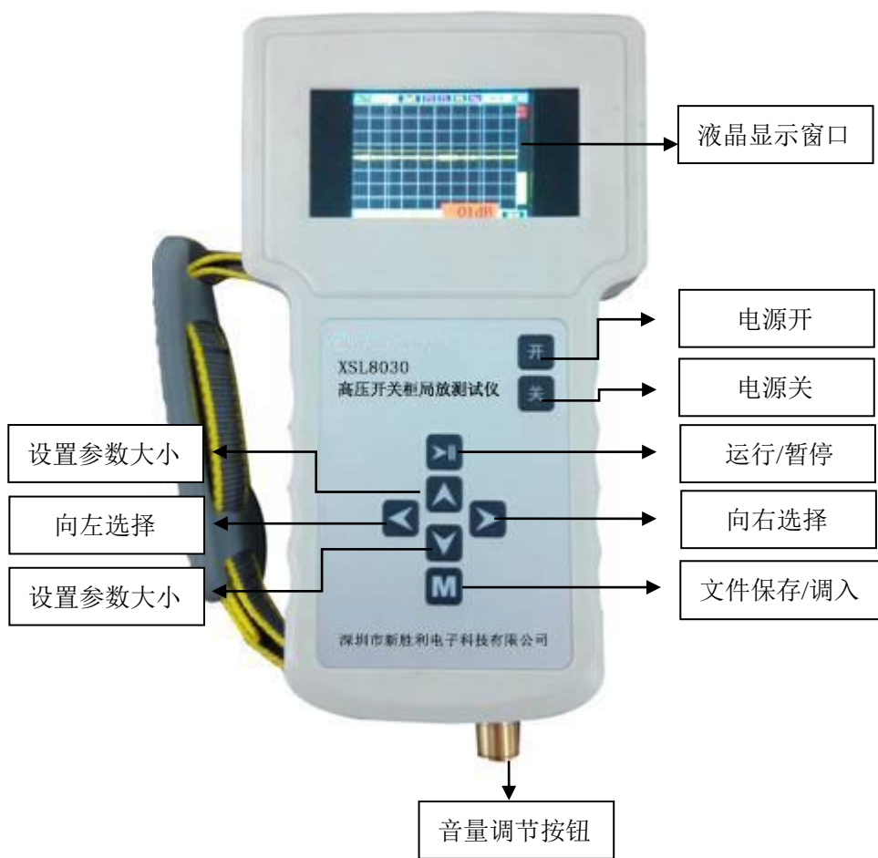
主机正面图
