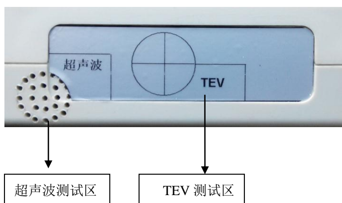
主机顶端图
