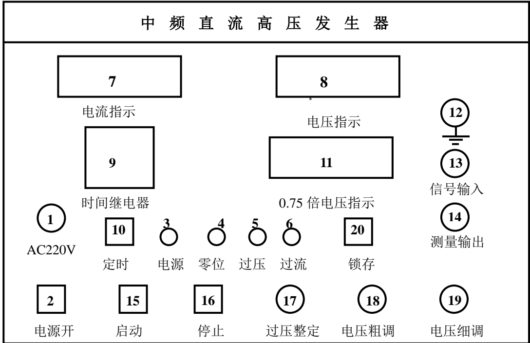
图 2. 控制箱面板布置图
