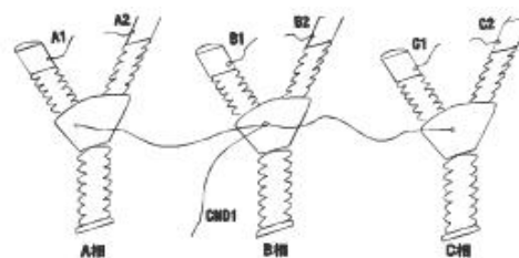
六断口信号线的连接
