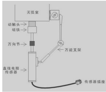
安装示意图
