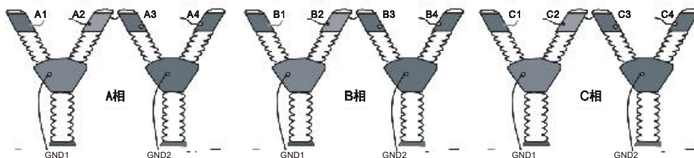
十二断口信号线的连接
