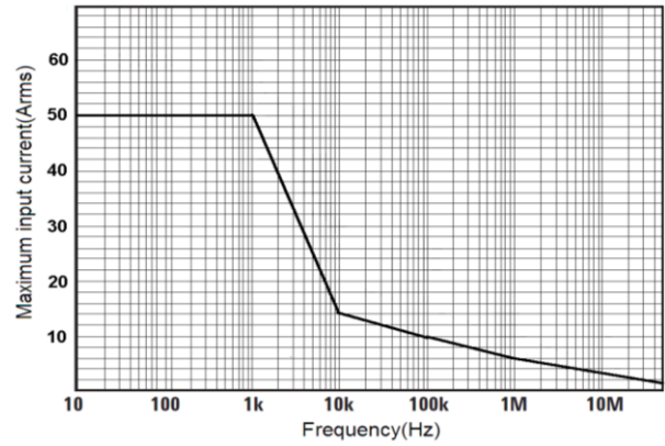
图 5 HCP8050 最大测量电流 VS 频率曲线 (超过该曲线所示最大电流连续使用会导致探头烧毁)
