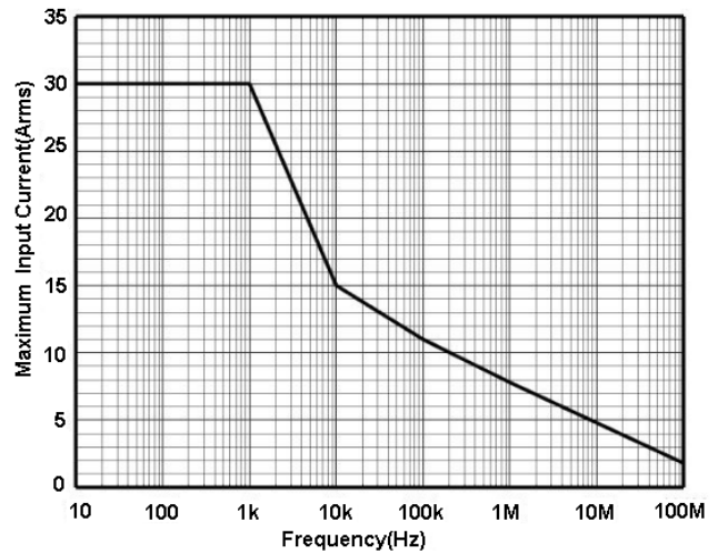
图 2.b HCP8030D 最大测量电流 VS 频率曲线
