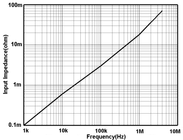
图 15 HCP8500 输入阻抗 VS 频率曲线
