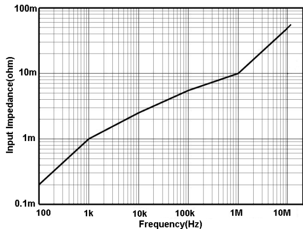
图 9 HCP8150 输入阻抗 VS 频率曲线
