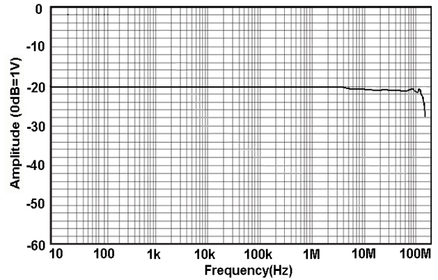
图 1 .b HCP8030D 幅频曲线
