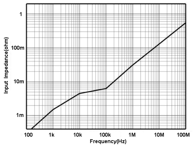
图 3.b HCP8030D 输入阻抗 VS 频率曲线
