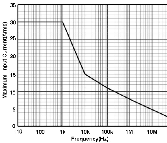
图 2.a HCP8030 最大测量电流 VS 频率曲线
