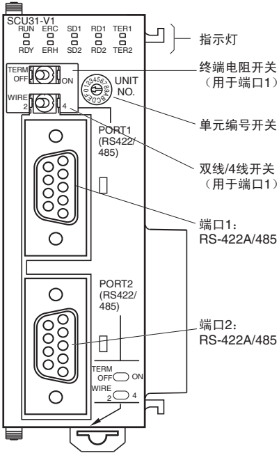
CJ1W-SCU31-V1
