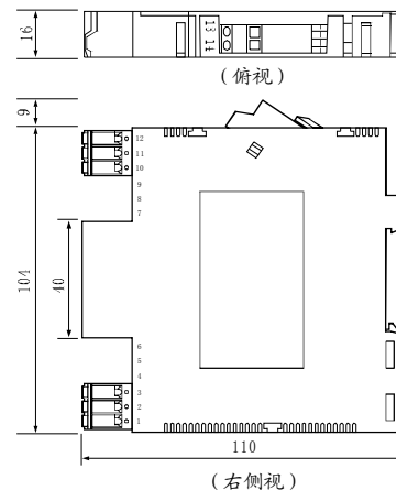
（右侧视）
