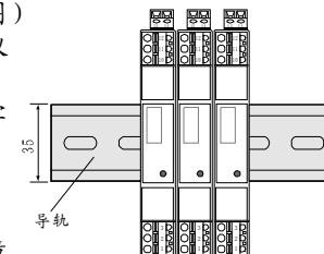
垂直安装示意图
