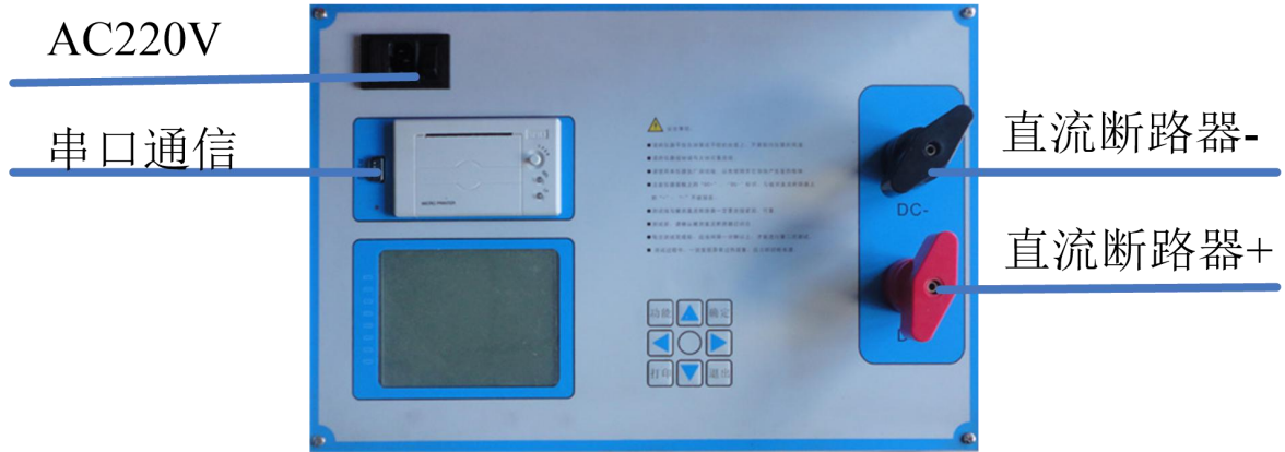
图 1 接线示意图
